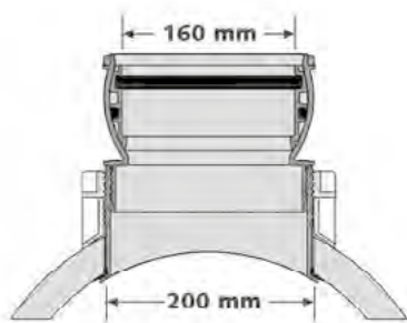
Przylącze siodłowe CONNEX DN/OD 160/200
