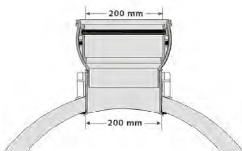
Przylącze siodłowe CONNEX DN/OD 200/200
